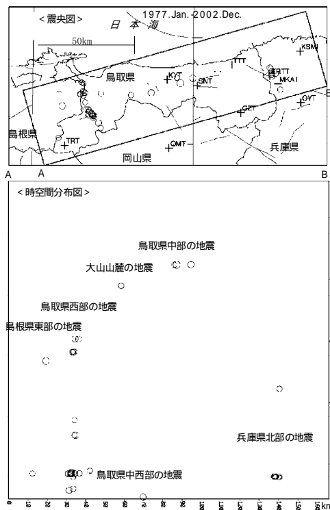
図1 山陰の地震活動 (M ≥ 4.5) (上図：震央図、下図：時空間分布図)
