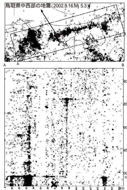
図2 山陰の地震活動 (M 0.0) (上図：震央図、下図：時空間分布図)
