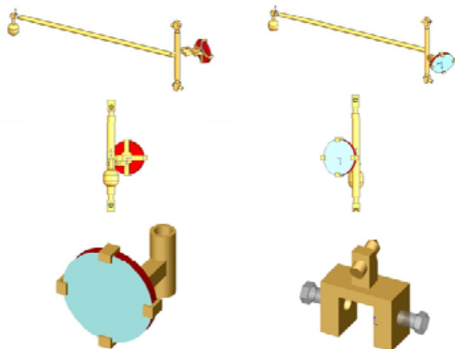
図7 センサー部3種
