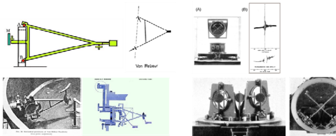
図1 構造原理と傾斜計写真
