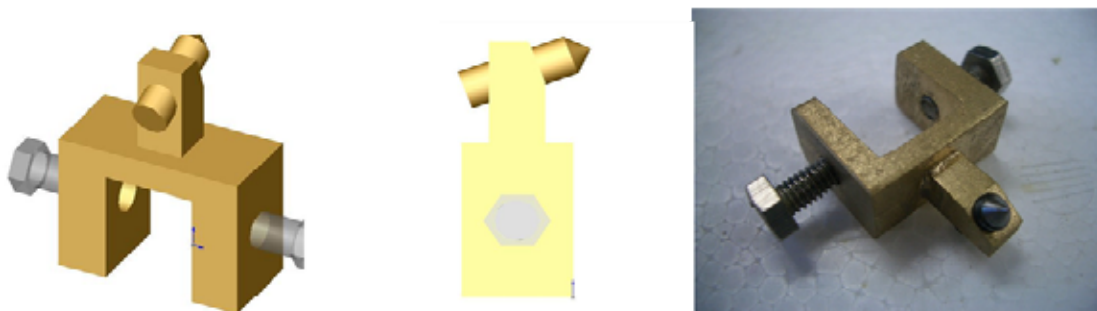
図6 下部支持金具
