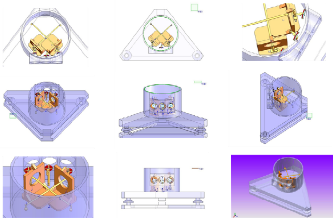
図8 3D/CADで表示のドイツ傾斜計模式図
