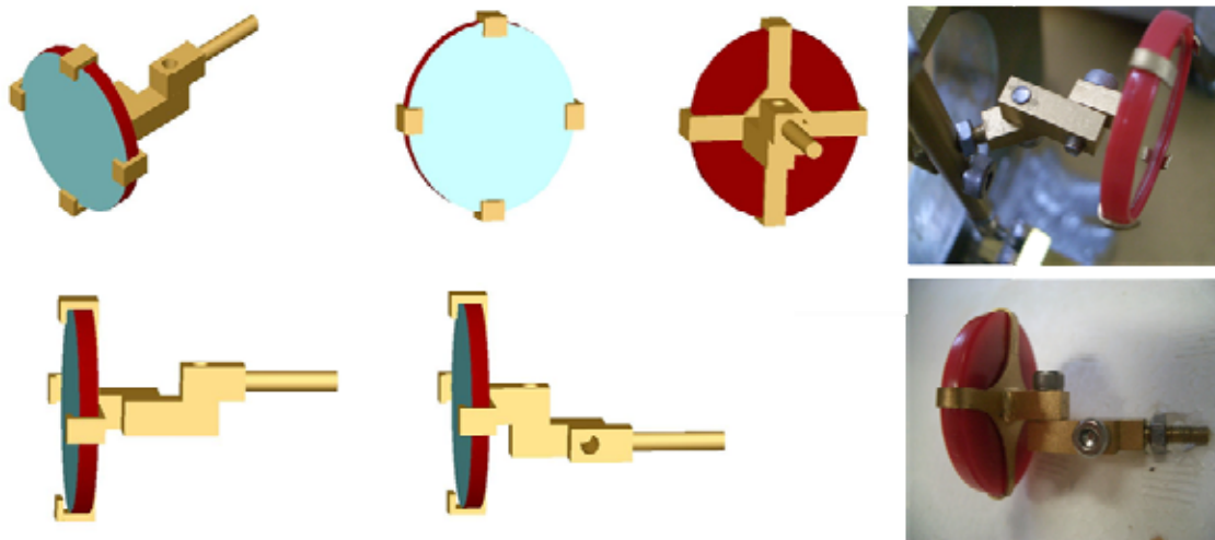
図4 NS・EWミラー支持金具
