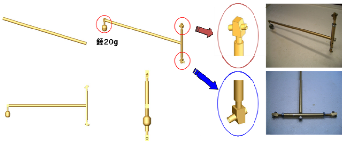
図 2 NS・EW成分の振子
