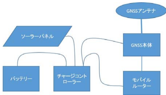
図 2 機器構成図
