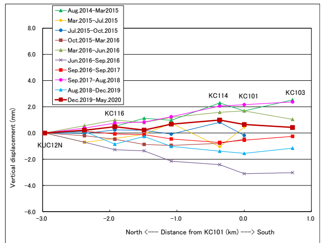
図 3. 水準測量結果。最新の測量は、2020 年 5 月 12 日-13 日に実施 (測量区間: KUC12N~KC103)。路線最北部の KUC12N を基準。2019 年 12 月 9 日-10 日 (前回測量) ~2020 年 5 月 12 日-13 日の期間 (図中の茶色太線)、変動量はそれほど大きくないが、路線南部に向かって地盤隆起傾向を示している (KC114 で 1.0 mm)。
