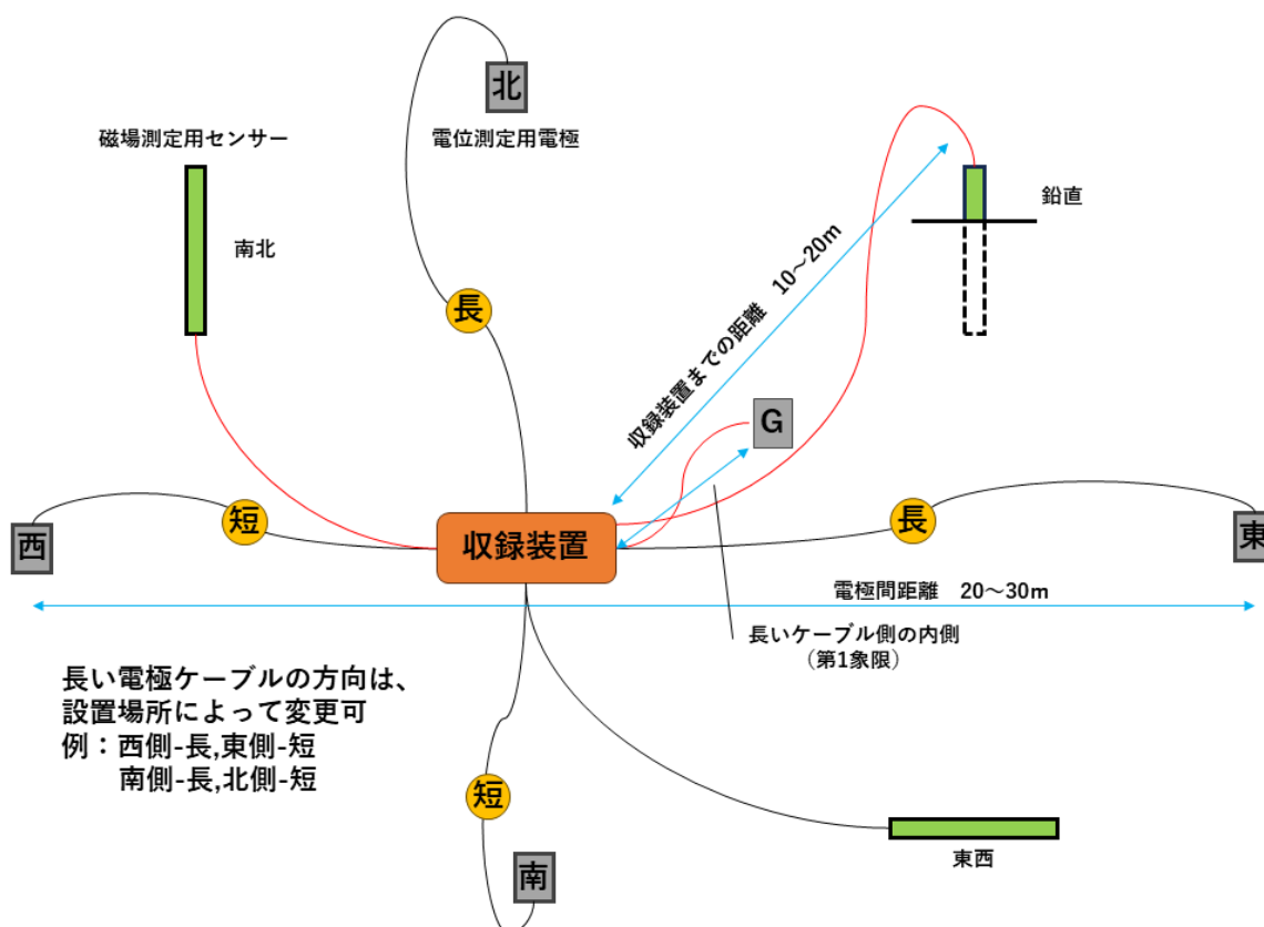
図1 観測機器の配置
